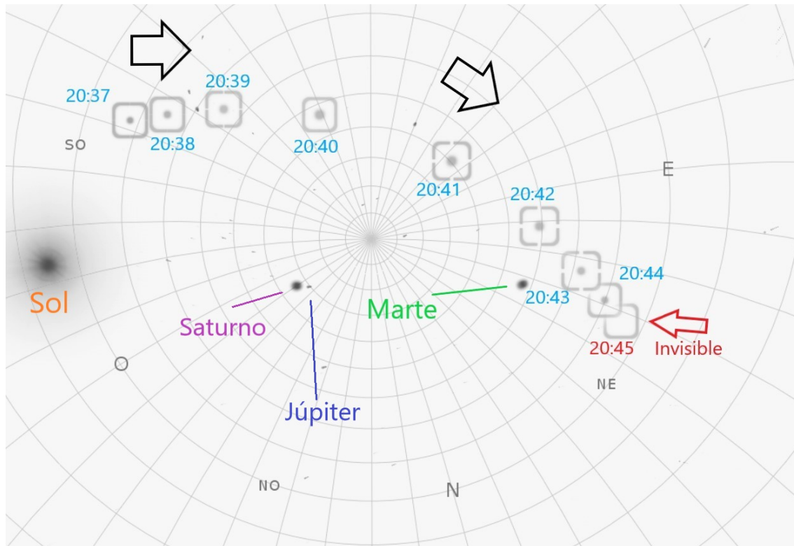
Figura 4. Sobrevuelo de la Estación Espacial Internacional del 5 de noviembre de 2020. Flechas negras señalan la dirección del desplazamiento.
